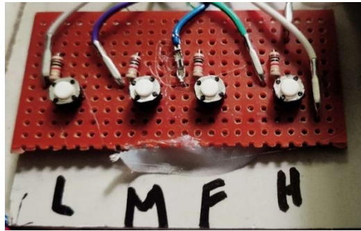
Fig. 14. Manual switches
