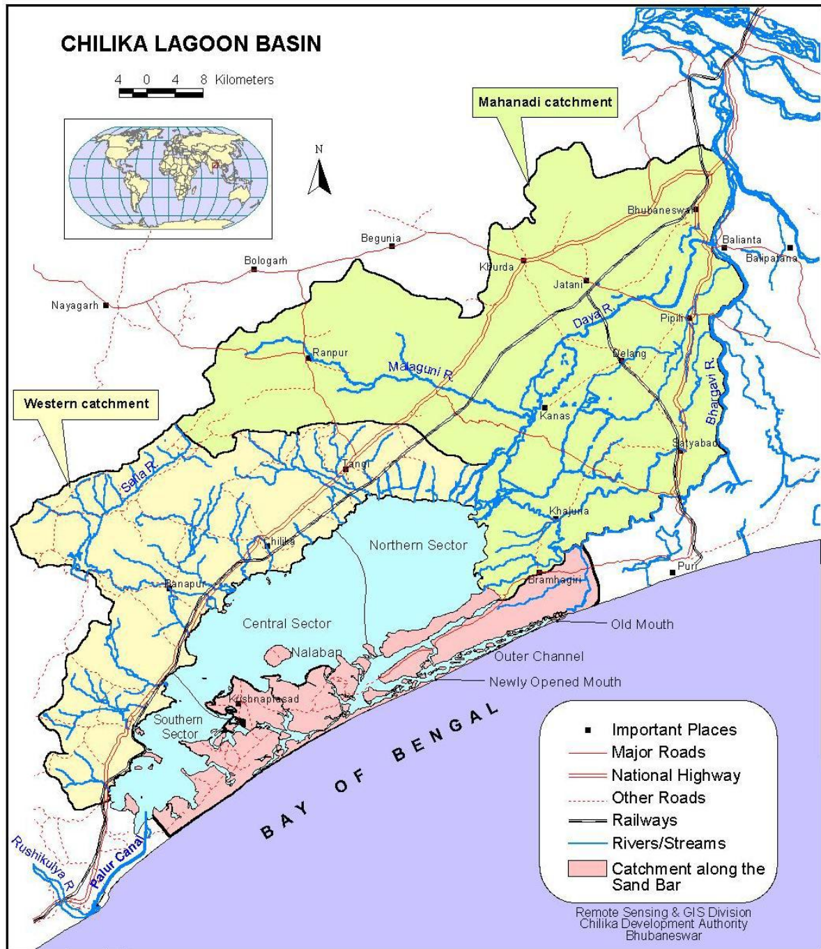
Fig. 1. Map of Chilika Lake
